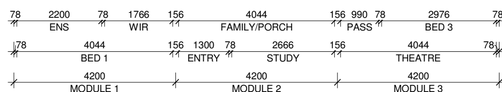
1 FLOOR PLAN 1 : 100
